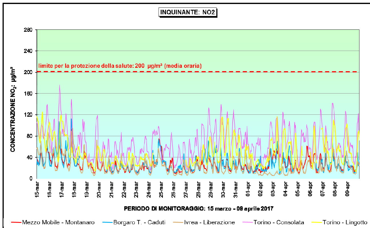
Figura 18 – \text{NO}_2 : confronto con i limiti di legge e con i dati di altre stazioni di monitoraggio
